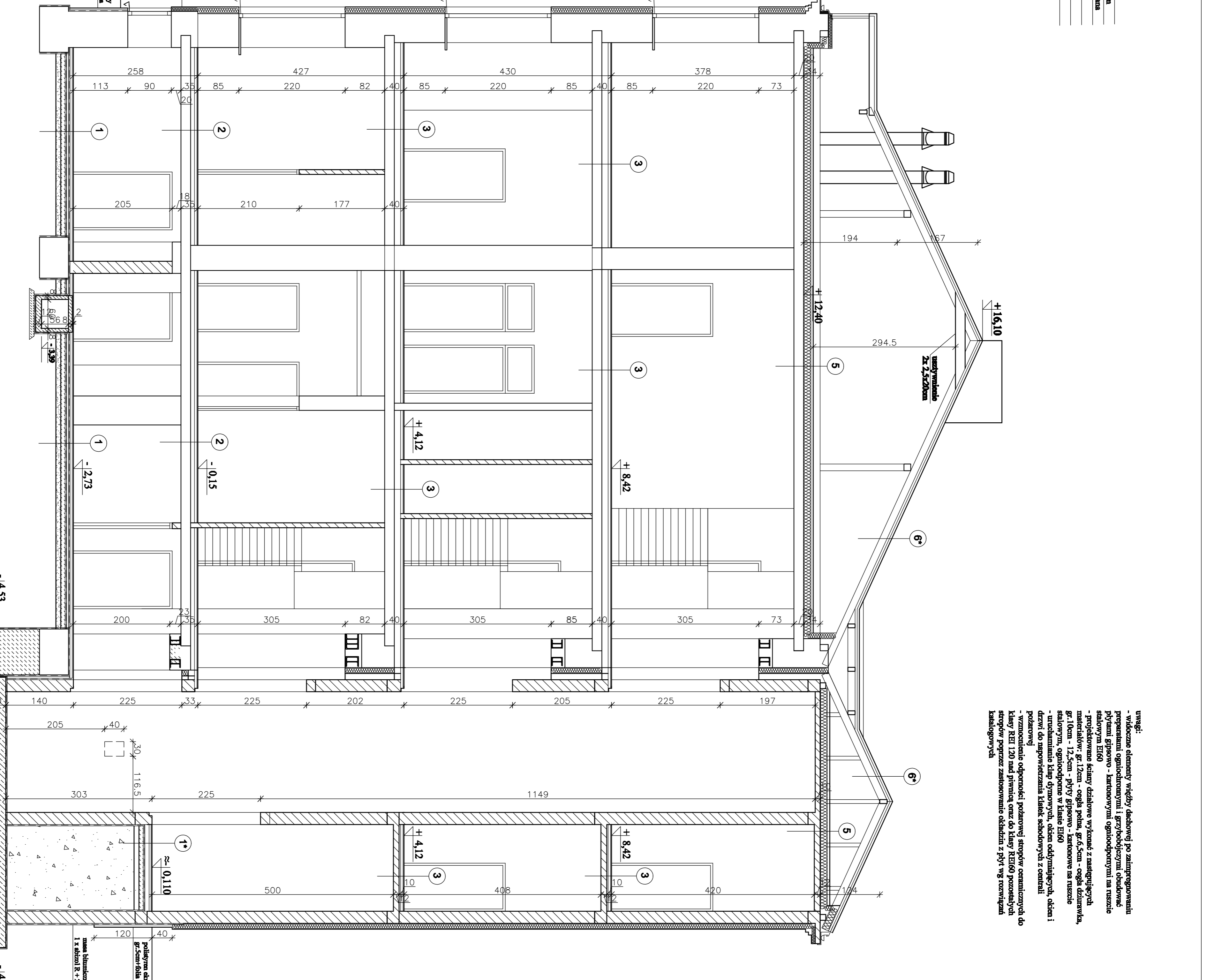
przekrój f-f
